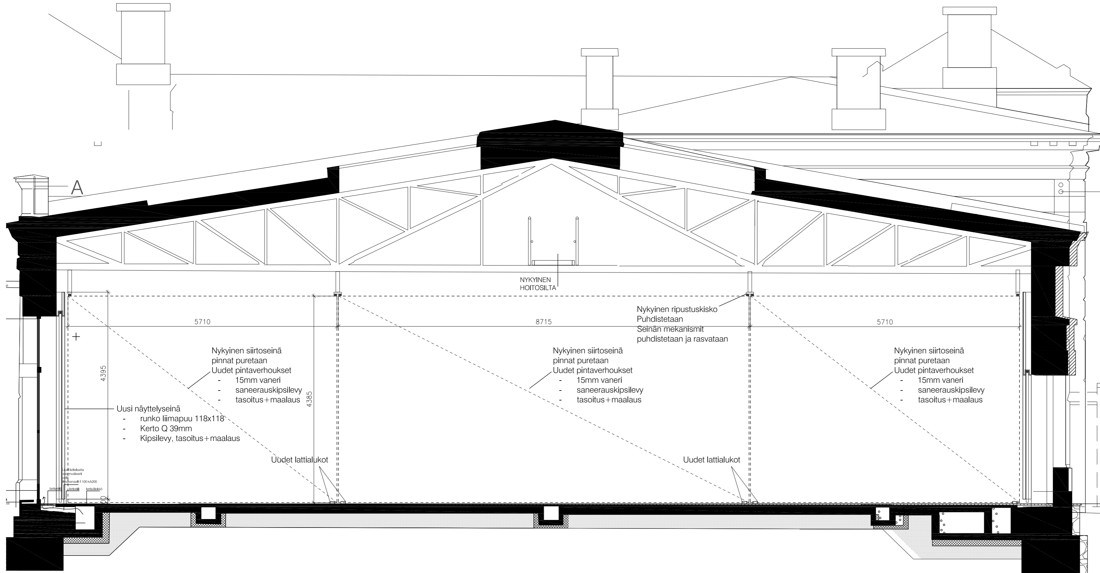
Leikkaus A-A, projektio siirrettävät näyttelyseinät 1:50
