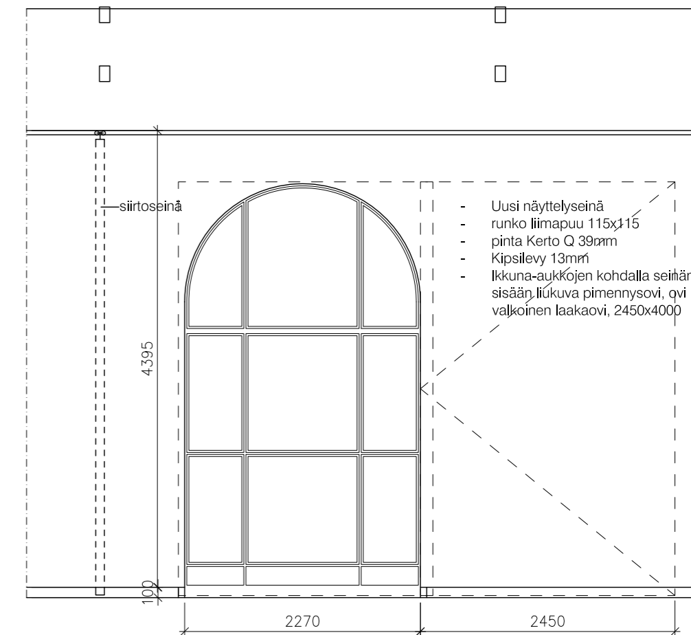
Projektio kiinteä näyttelyseinä 1:50
